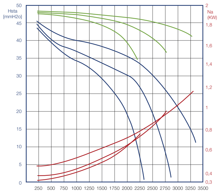
PORTATA - VOLUME FLOW Q (m 3 /h)
